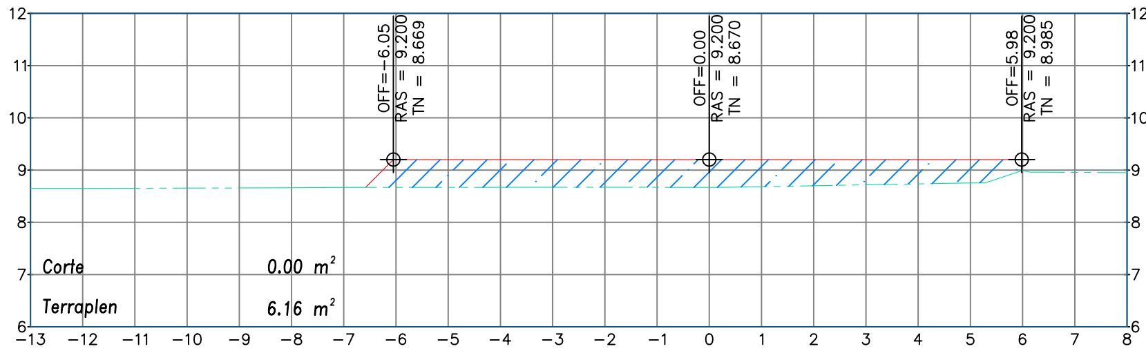
ESTACION 0+020.00 ESCALA: 1:100 EXAGERACIÓN VERTICAL: 1:1
