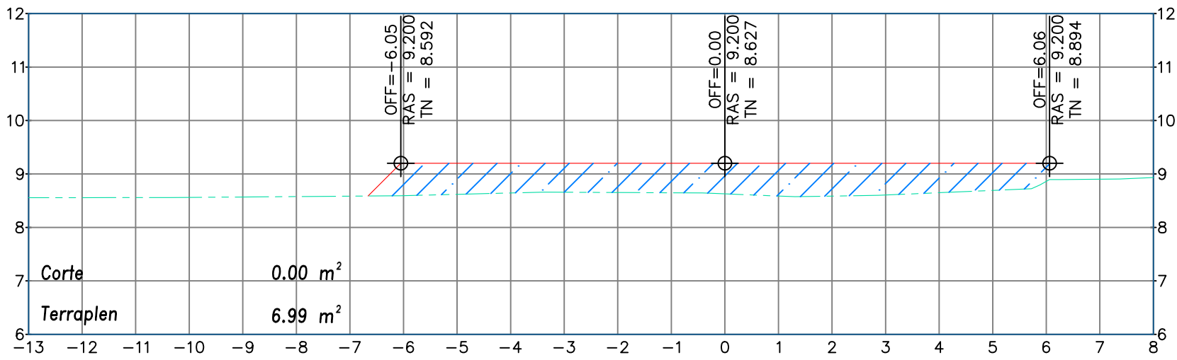
ESTACION 0+035.00 ESCALA: 1:100 EXAGERACIÓN VERTICAL: 1:1
