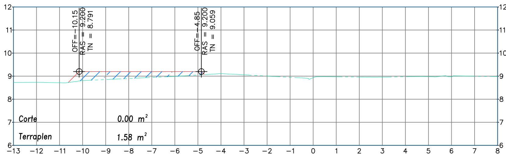
ESTACION 0+001.27 ESCALA: 1:100 EXAGERACIÓN VERTICAL: 1:1
