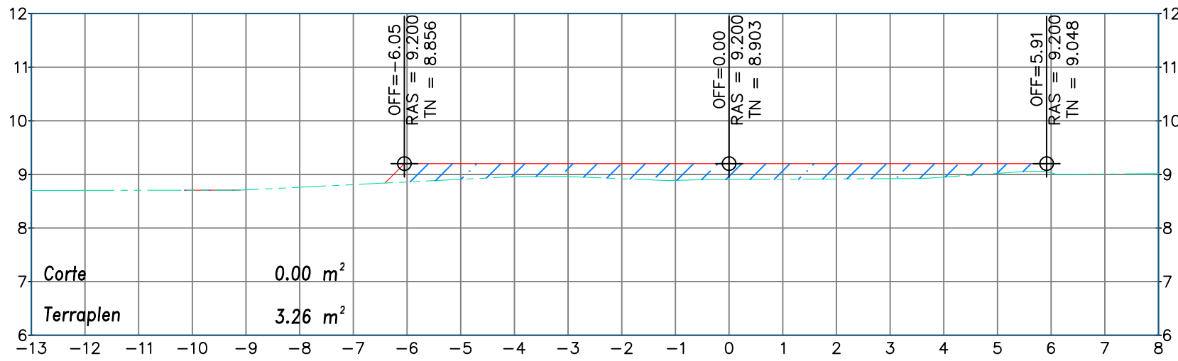
ESTACION 0+007.05 ESCALA: 1:100 EXAGERACIÓN VERTICAL: 1:1
