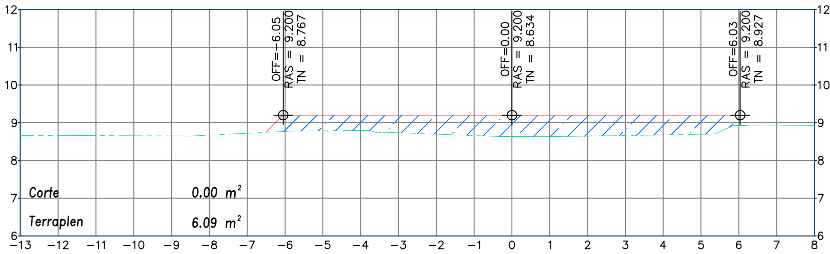
ESTACION 0+030.00 ESCALA: 1:100 EXAGERACIÓN VERTICAL: 1:1
