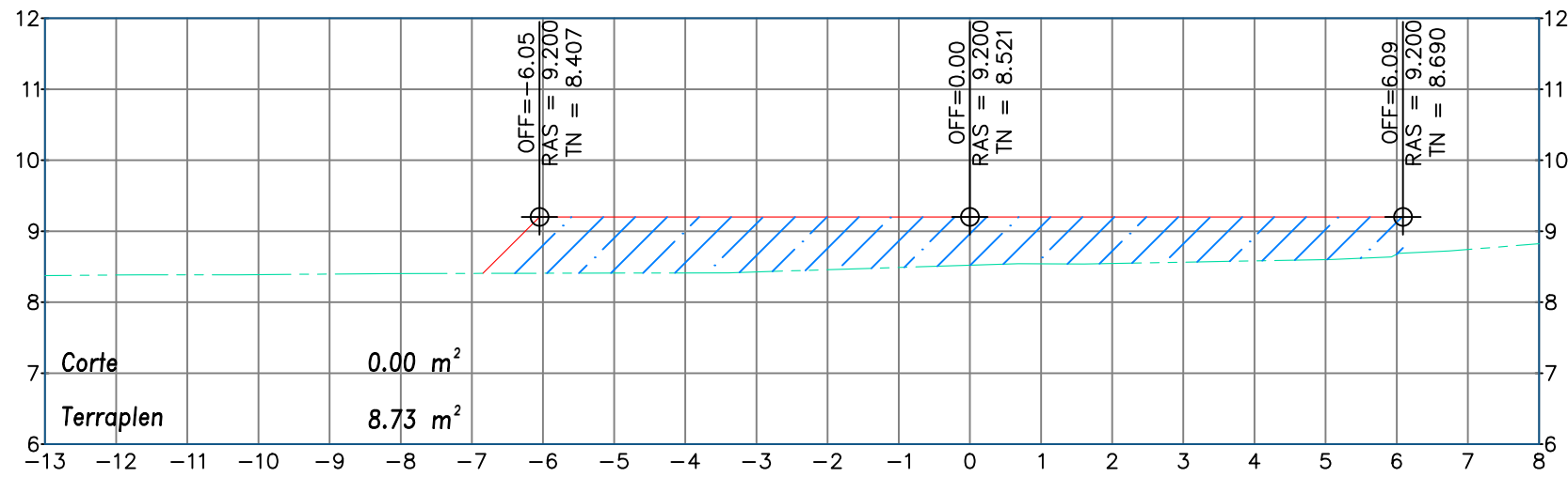
ESTACION 0+040.00 ESCALA: 1:100 EXAGERACIÓN VERTICAL: 1:1
