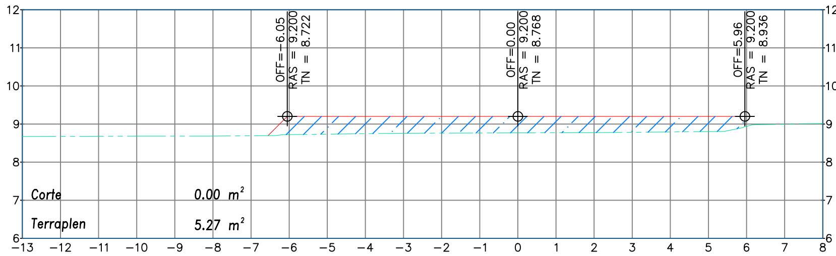
ESTACION 0+015.00 ESCALA: 1:100 EXAGERACIÓN VERTICAL: 1:1
