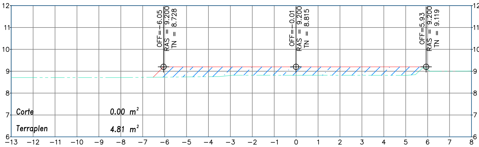
ESTACION 0+010.00 ESCALA: 1:100 EXAGERACIÓN VERTICAL: 1:1
