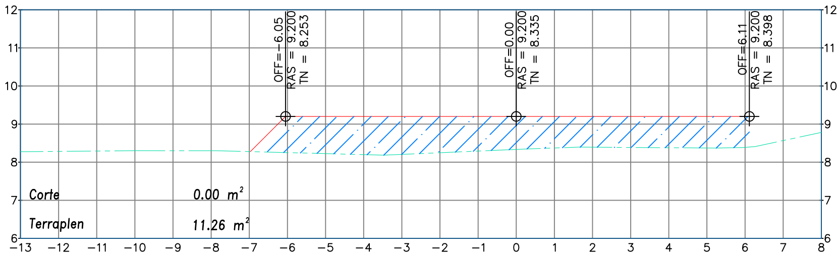
ESTACION 0+045.00 ESCALA: 1:100 EXAGERACIÓN VERTICAL: 1:1
