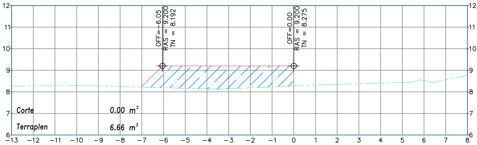
ESTACION 0+046.40 ESCALA: 1:100 EXAGERACIÓN VERTICAL: 1:1
