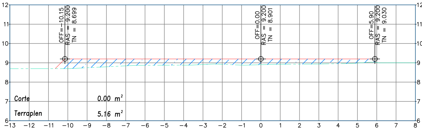
ESTACION 0+005.00 ESCALA: 1:100 EXAGERACIÓN VERTICAL: 1:1
