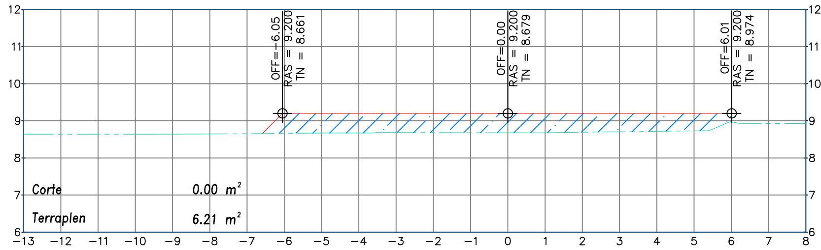
ESTACION 0+025.00 ESCALA: 1:100 EXAGERACIÓN VERTICAL: 1:1
