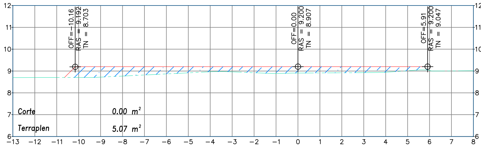
ESTACION 0+006.56 ESCALA: 1:100 EXAGERACIÓN VERTICAL: 1:1
