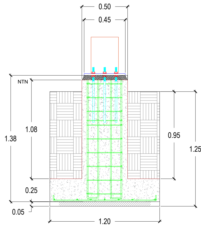
ZAPATA ZA-1 DE 1.20X 1.20 PLANTILLA VAR 1/2 @ 15 CM
