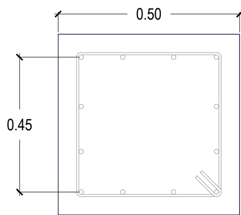
DA-1 0.50 X 0.50 M 12 var 1/2 EST #2 @15 CM
