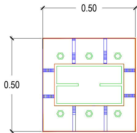
PB-1 e 3/4" 0.50 X 0.50 M ANCLA 6 VAR 3/4 PERFORACION PARA ANCLAS DE 3/4
